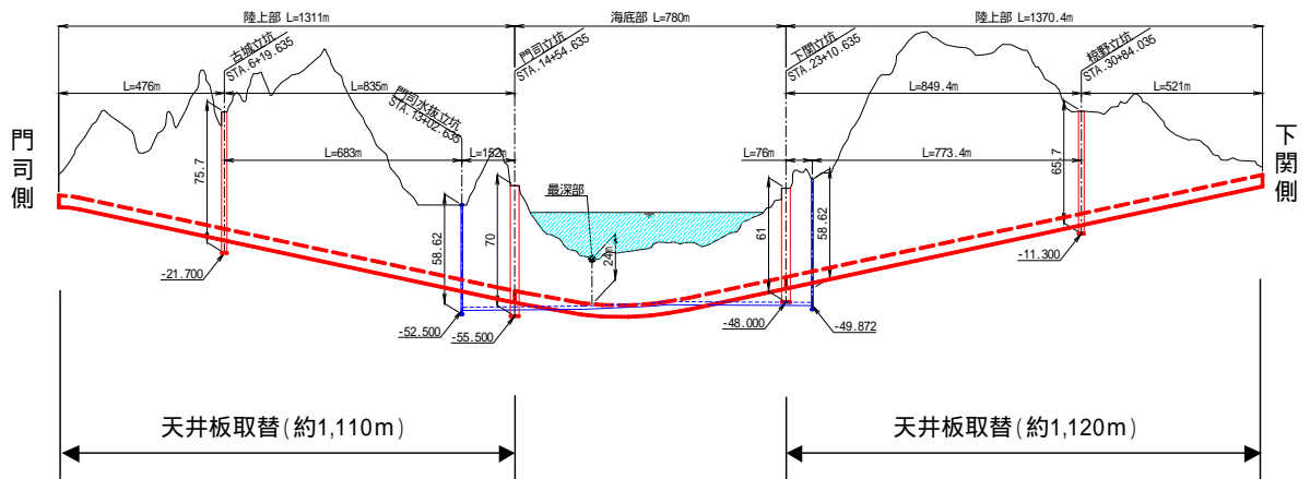
縦断面図
