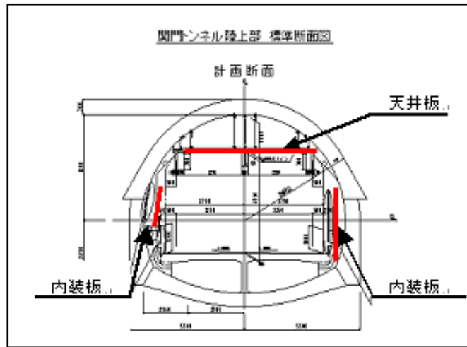
横断面図
