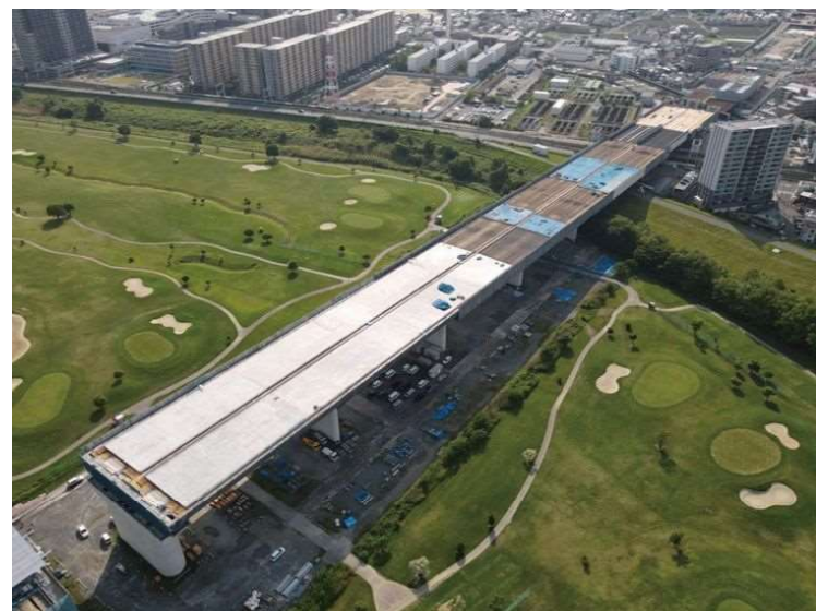
⑥ 橋梁上部工の施工を行っております。
