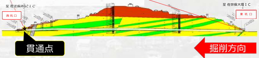
天神山トンネル縦断面図
