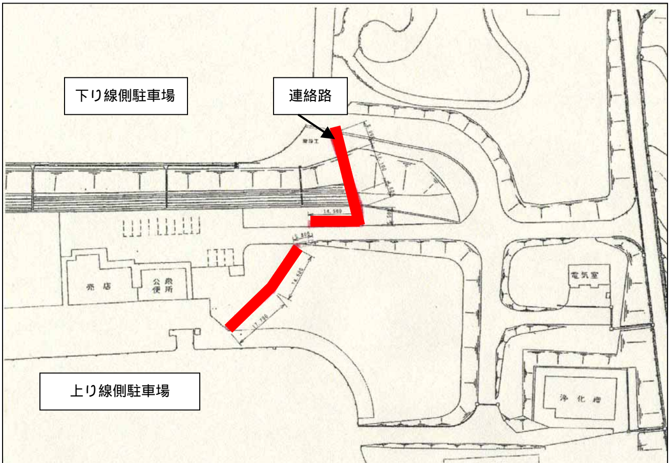
佐波川 S A 上下線連絡路位置図
