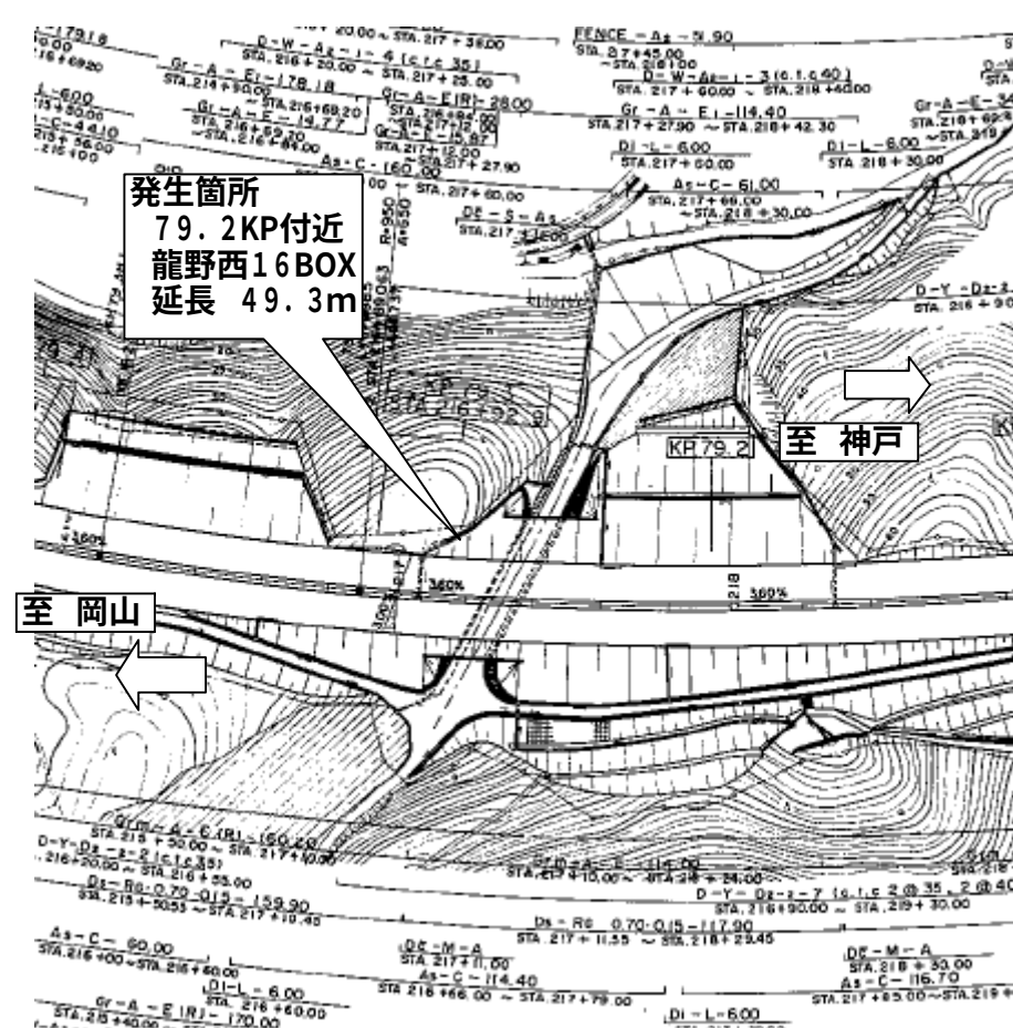
平面図
