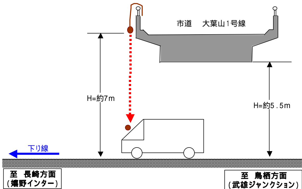
長崎自動車道 前山跨道橋 落下事象概要図
