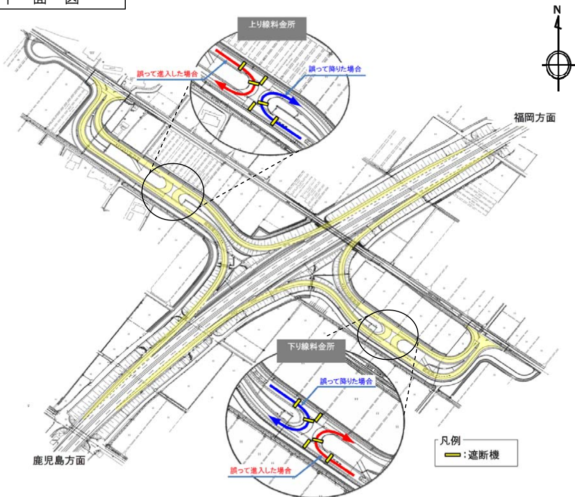
平面図
