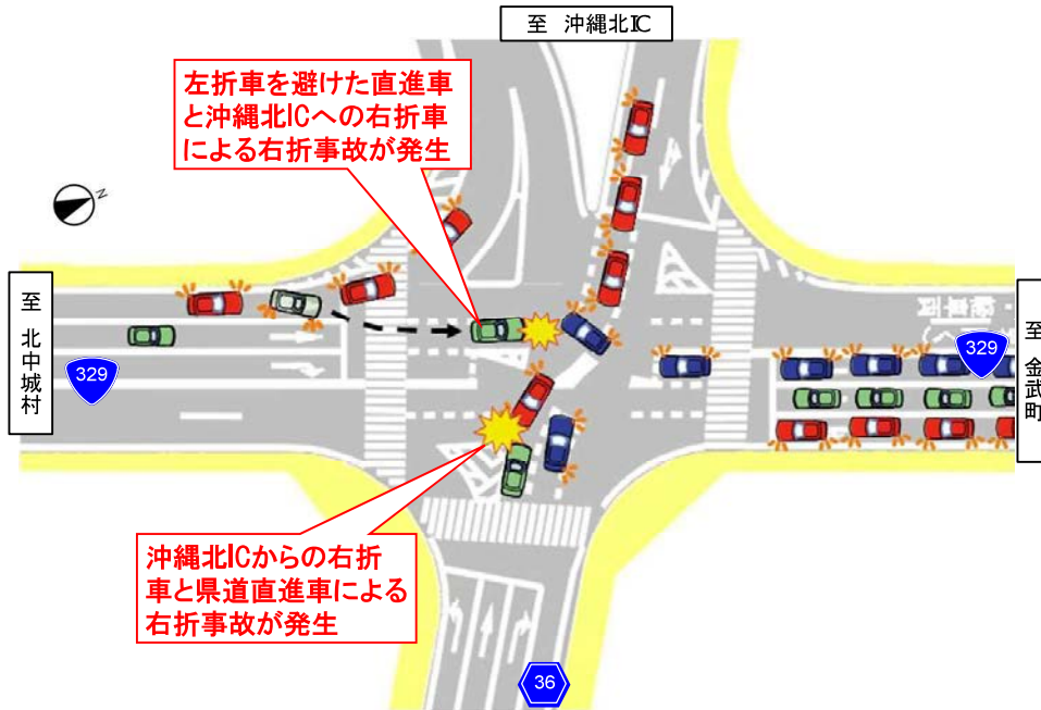
交差点流入部及び交差点内における人身事故内訳
