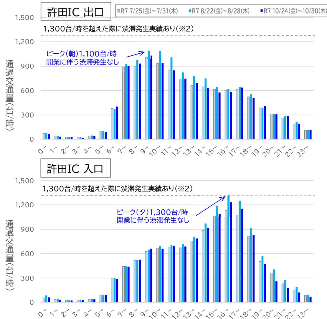
時間帯別通過交通量(許田料金所)【開業1か月後・3か月後の1週間平均】
