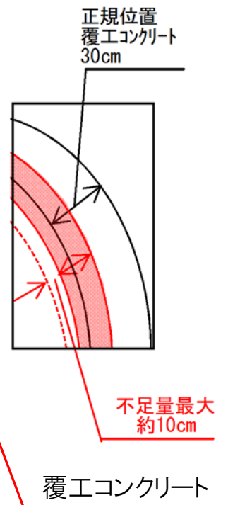
覆工コンクリート横断図
