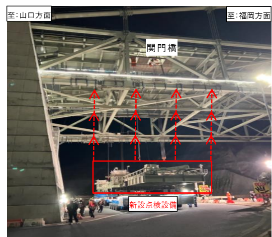
《(2)新設点検設備 吊上架設前》
