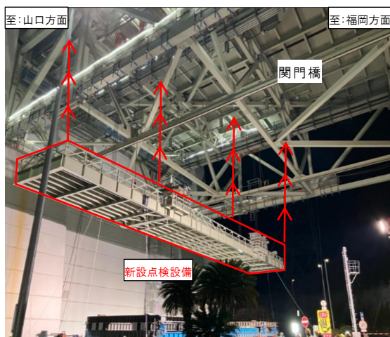
《(3)新設点検設備吊上架設中》
