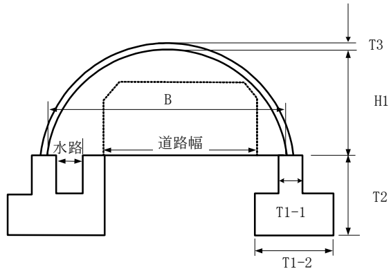
独立基礎タイプ(1)
