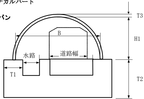
インバート付基礎
