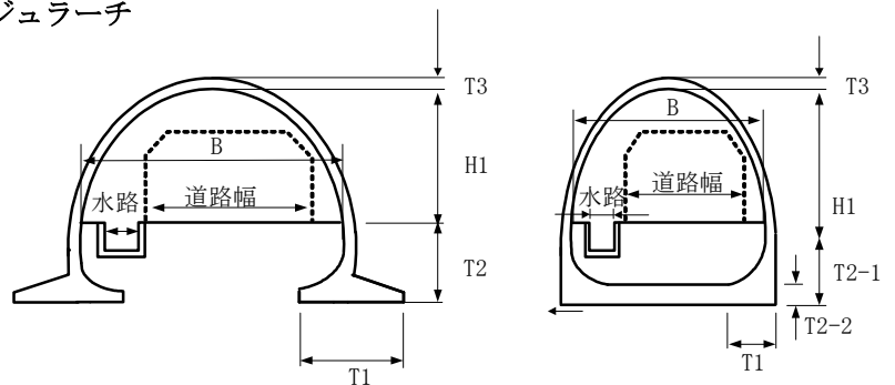
フーチングタイプ
